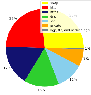
(c) CTU-13
