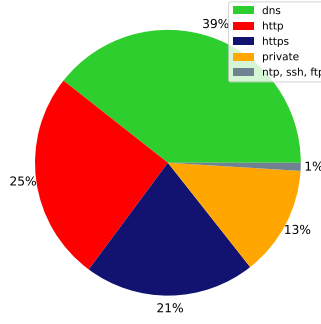
(d) CICIDS17
