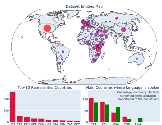
(h) kiSwahili
