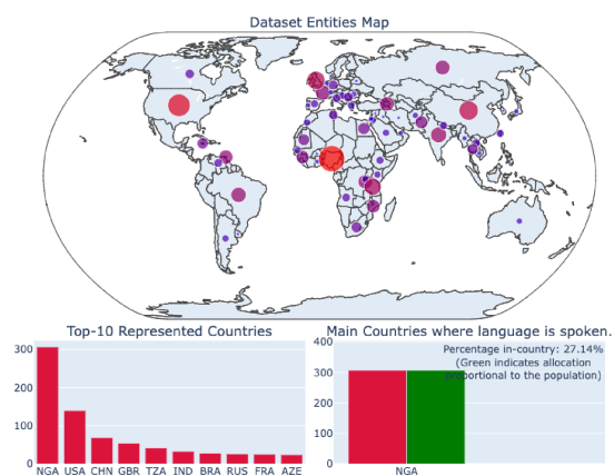
(j) Yoruba
