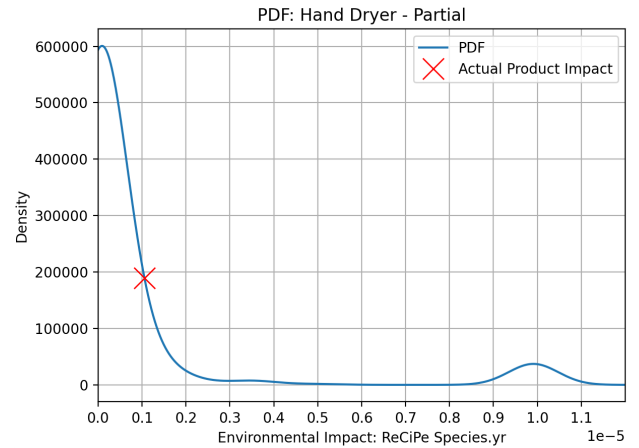
(d) Hand Dryer partial BOM probability density function
