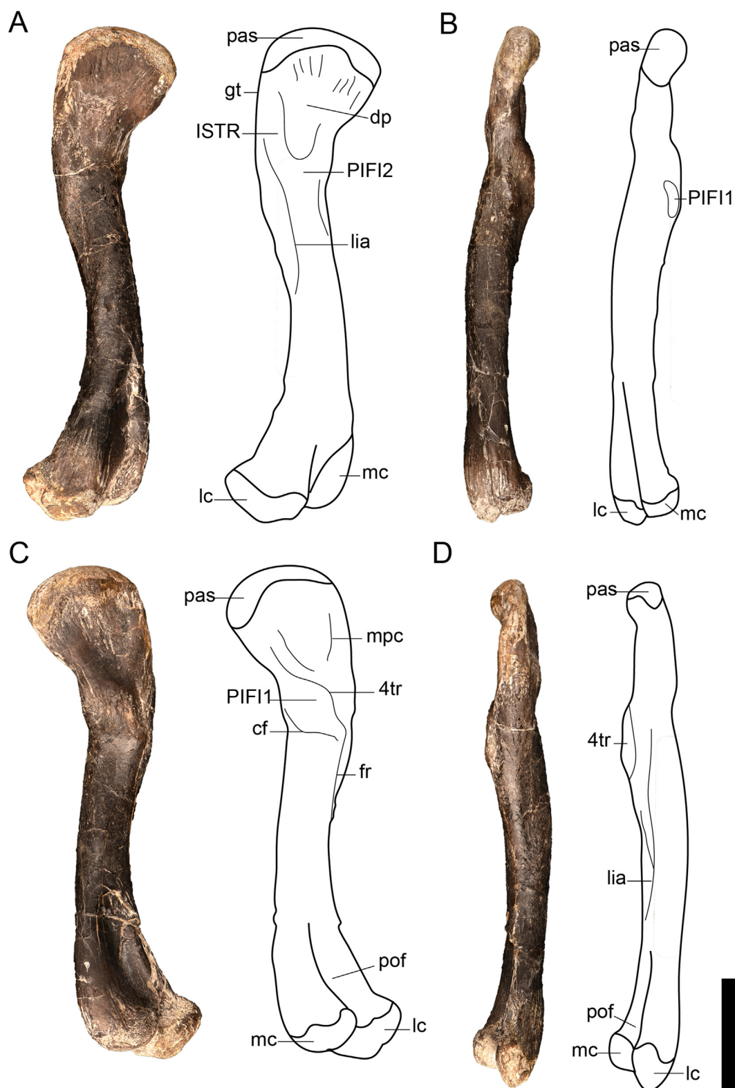
Fig. 13. Right femur of Yanjisuchus longshanensis gen. et sp. nov., holotype (YJDM 00009), in lateral (A), anterior (B), medial (C), and posterior (D) views. Scale bar = 3 cm.
