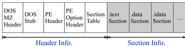
Fig. 2. The Structure of PE file format.
