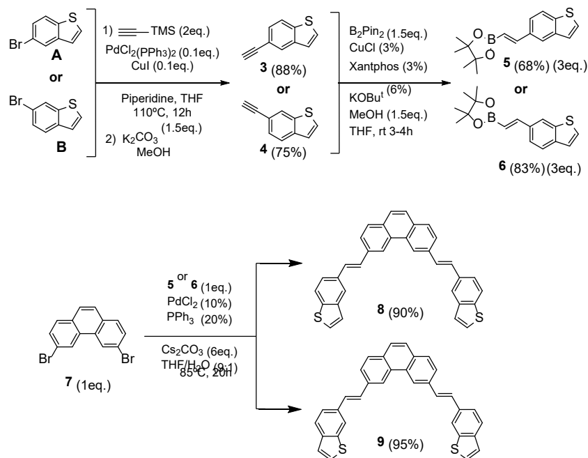
Scheme 1. Synthesis of 3,6- bis -( E )-2-(benzo[ b ]tiophen-5-yl)vinyl)phenanthrene ( 8 ) and 3,6- bis -( E )-2-(benzo[ b ]tiophen-6-yl)vinyl)phenanthrene ( 9 ).
