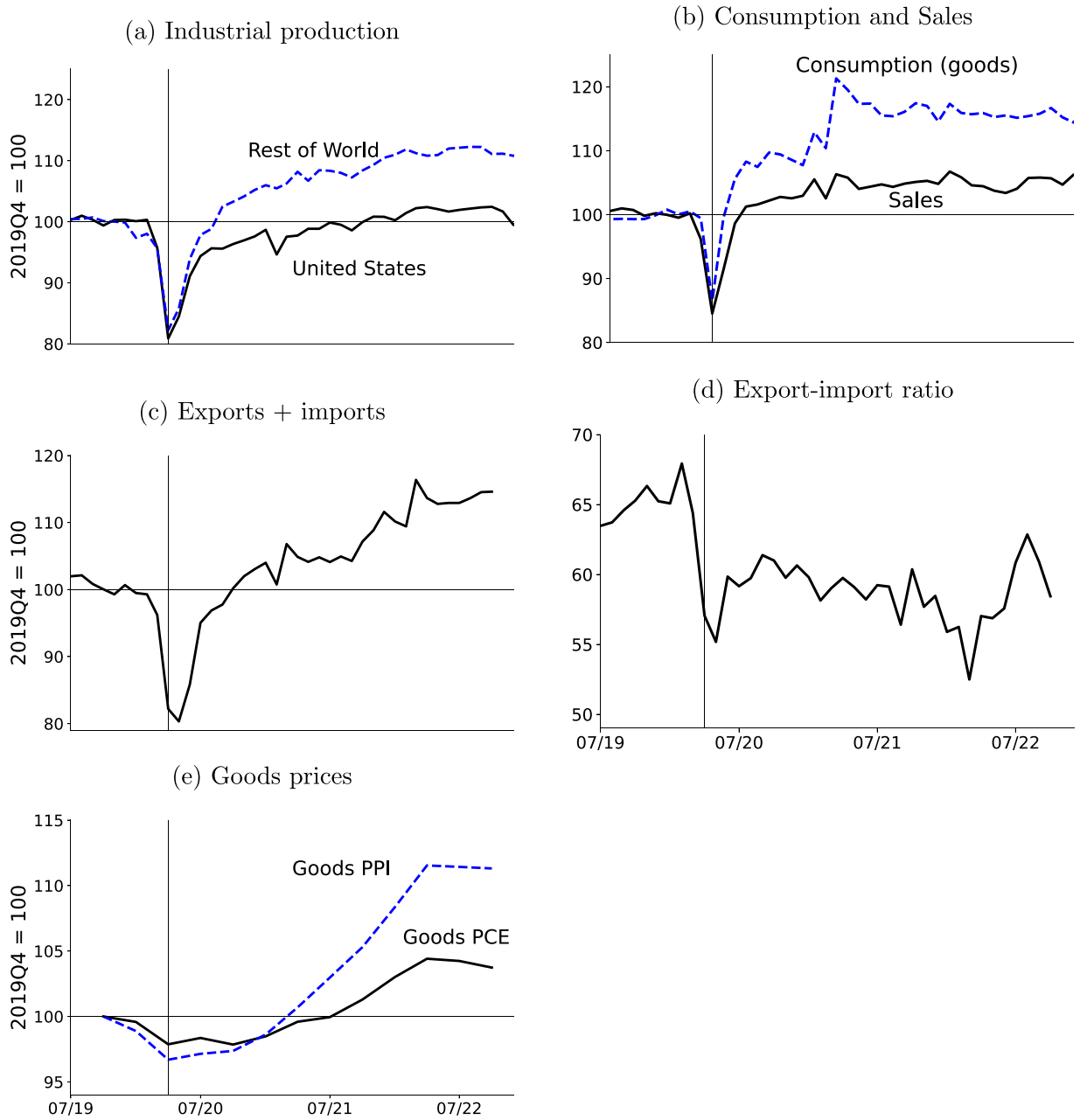
Fig. 8. Salient features.
