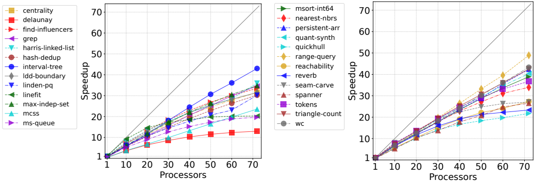
Fig. 7. Speedups
