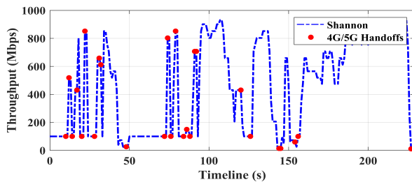
Fig. 4. [23] 4G/5G NR Shannon throughput
