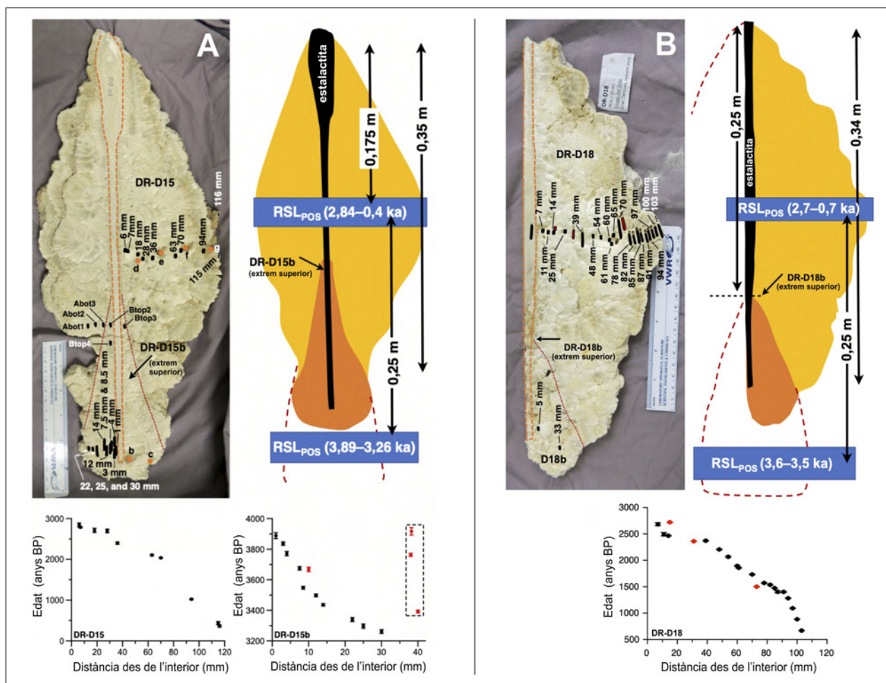
Figura 11: Els POS compostos DR-D15/15b (A) i DR18/18b (B) de les Coves del Drac (Manacor). Vista en secció dels espeleotemes amb la localització de les submostres extreptes per a les datacions U-Th, i interpretació morfogenètica que es deriva (RSL POS = nivells marins relatius deduïts dels POS i les seves edats). S'han identificat dos nivells marins successius, separats per una pujada de 25 cm del nivell de la Mediterrània ocorreguda entre 3,26 i 2,84 ka BP. Les gràfiques de la banda inferior de la figura representen la cronologia de la deposició dels POS; els símbols vermells corresponen a datacions de capes contaminades o alterades, que han subministrat edats sense coherència estratigràfica (Modificat a partir d'ONAC et al., 2022).
