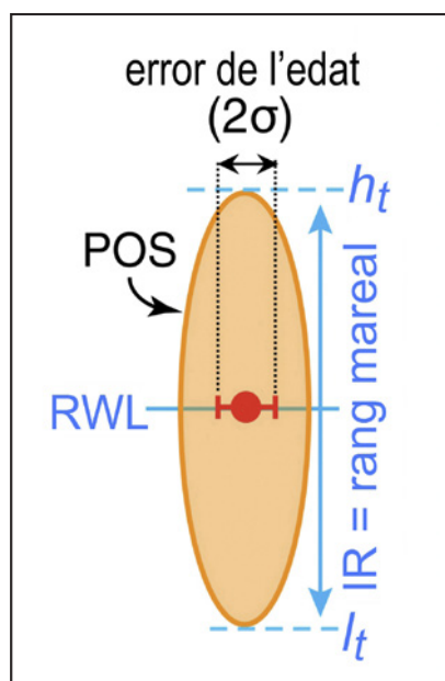
Figura 6: Els espeleotemes freàtics holocènics de Mallorca. Representació esquemàtica d'un POS, on s'observa com la part més gruixuda (RWL) correspon a la posició mitjana del nivell marí durant el període de formació del POS. IR = indicative range; h_t = marea alta; l_t = marea baixa; vegeu informacions addicionals en el text (Modificat a partir d'ONAC et al., 2022). Figure 6: Holocene POS from Mallorca. Schematic representation of the indicative meaning of POS. The thickest part corresponds to the reference water level (RWL), which was the position of mean sea level for the period of POS formation. IR = indicative range; h_t = high tide; l_t = low tide; see additional information in the text (Modified from ONAC et al., 2022).
