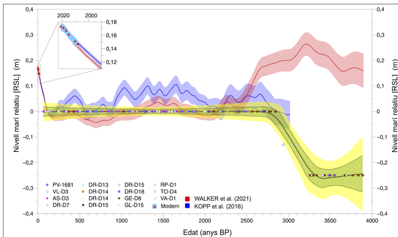
Figura 14: El nivell marí relatiu (RSL) a Mallorca durant l'holocè final, segons les dades aportades pels espeleotemes freàtics. El RSL romangué estable a -0,25 m entre \sim 3,89 i \sim 3,26 ka BP i, després d'una ràpida pujada, es va establir en el nivell marí preindustrial els darrers \sim 2,84 ka (les àrees acolorides en verd i en grog denoten, respectivament, els intervals de credibilitat del 67 i del 95%). Les corbes blava i vermella mostren el nivell marí global (GMSL) en relació a l'any 1900 segons KOPP et al. (2016) i WALKER et al. (2021). Els cercles i els rombes assenyalen, respectivament, els POS analitzats a la University of New Mexico i a la Universität Bern. El requadre superior recull la posició del nivell marí relatiu, mesurada a tres cavitats des del 2008 (Modificat a partir d'ONAC et al., 2022).
