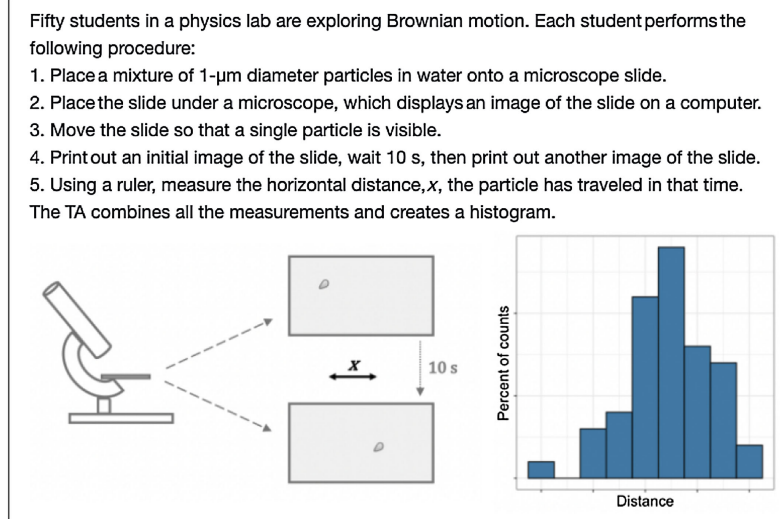
(b) Brownian motion scenario
