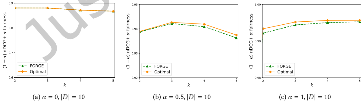
Fig. 11. FORGE vs optimal brute-force algorithm.
