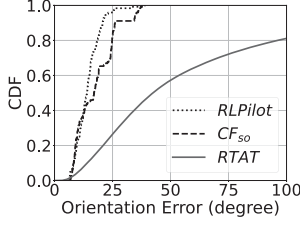
Fig. 8. Original dataset.
