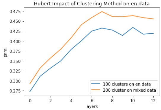
(d) 100 monolingual vs. 200 mixed units, evaluated on English data
