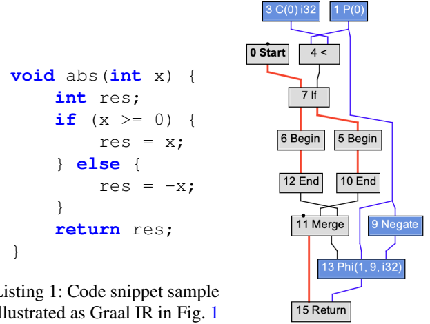
Fig. 1: Visualized Graal IR
