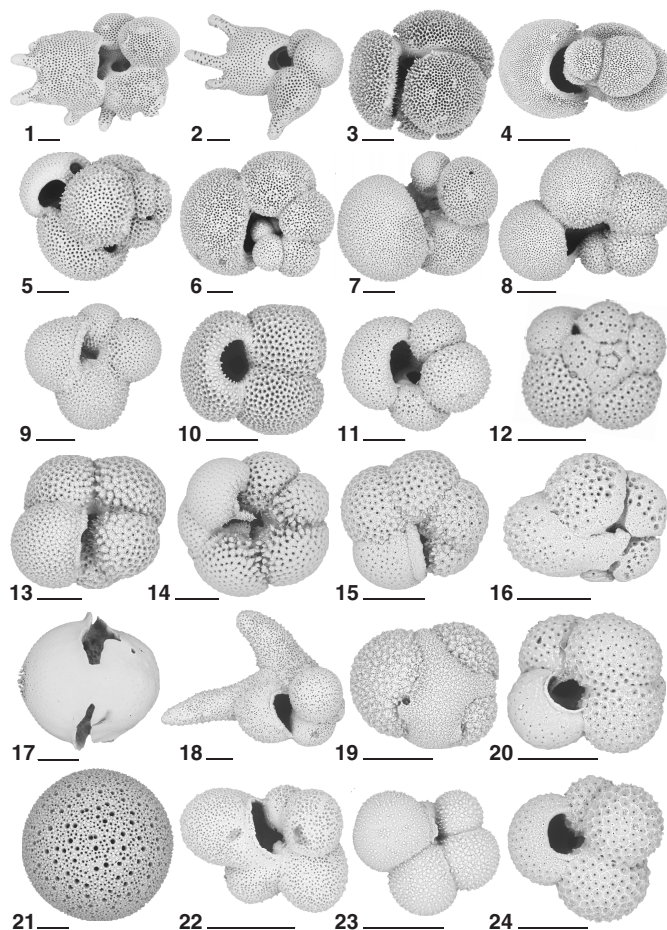
Figure F22. Planktonic foraminifers, Hole U1474A. Scale bars = 100 \mu m. 1, 2. Globigerinoides fistulosus (8H-6, 70–72 cm). 3. Globigerinoides conglobatus (3H-4, 70–72 cm). 4. Globigerinella siphonifera (2H-6, 70–72 cm). 5. Globigerinoides ruber (pink) (1H-4, 70–72 cm). 6. G. siphonifera (1H-4, 70–72 cm). 7. Globigerinella obesa (1H-4, 70–72 cm). 8. Globigerinella calida (1H-4, 70–72 cm). 9. Globigerina falconensis (7H-7, 70–72 cm). 10. G. ruber (white) (1H-4, 70–72 cm). 11. Globigerina bulloides (1H-4, 70–72 cm). 12. Turborotalita quinqueloba (1H-4, 70–72 cm). 13. Neogloboquadrina pachyderma (dextral) (1H-4, 70–72 cm). 14. Neogloboquadrina dutertrei (1H-4, 70–72 cm). 15. Neogloboquadrina acostaensis (7H-4, 70–72 cm). 16. Turborotalita quinqueloba (1H-4, 70–72 cm). 17. Spheroidinella dehiscens (1H-4, 70–72 cm). 18, 22. Beela digitata (2H-6, 70–72 cm). 19. Globigerinita glutinata (1H-4, 70–72 cm). 20. Globoturborotalita rubescens (1H-4, 70–72 cm). 21. Orbulina universa (1H-4, 70–72 cm). 23. Tenuitella anfracta (27H-1, 70–72 cm). 24. Globoturborotalita tenellus (3H-4, 70–72 cm).
