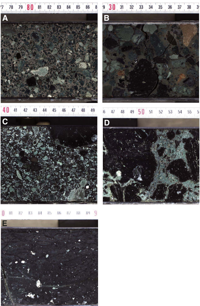
Figure F4. Lithostratigraphic subunits, Hole M0077A. A. Subunit 2A (suevite; 40R-2). B. Subunit 2B (suevite; 72R-2). C. Subunit 2C (suevite; 84R-3). D. Subunit 3A (impact melt rock; 88R-3). E. Subunit 3B (impact melt rock; 94R-3).
